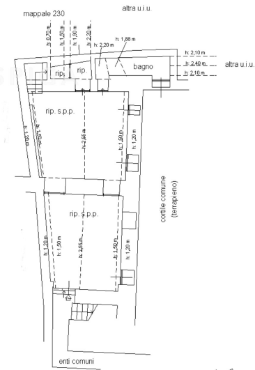
PIANO PRIMO INTERRATO
